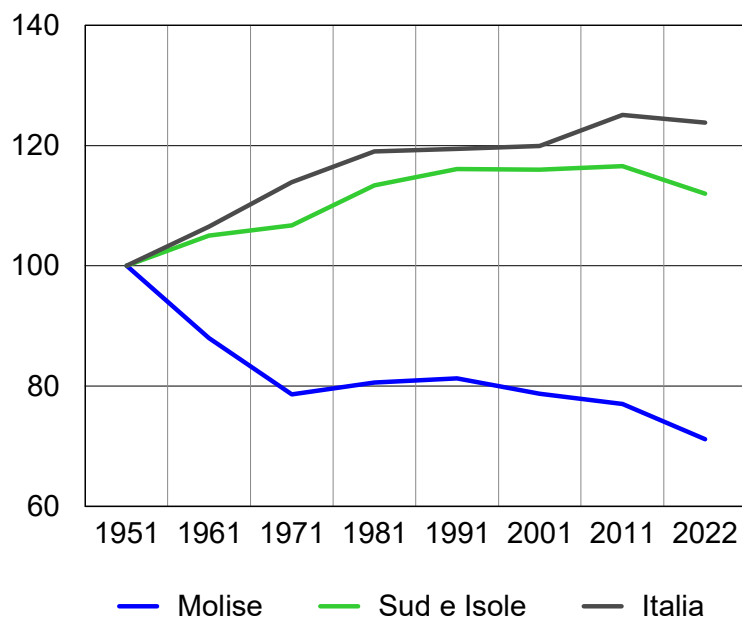
Popolazione tra il 1951 e il 2022
